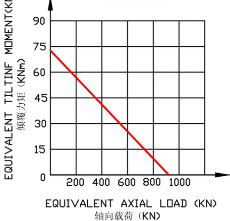
SIZE 341 MOMENT LOAD CHART 341 承载能力曲线图
